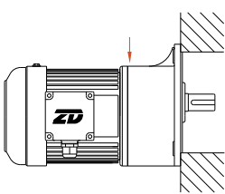
Q1 出气孔方向 Air hold direction
