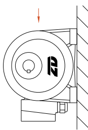
Q5 出气孔方向 Air hold direction
