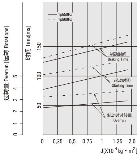
负载惯性质量 Load Inertia
